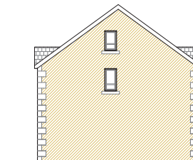
RHS ELEVATION
